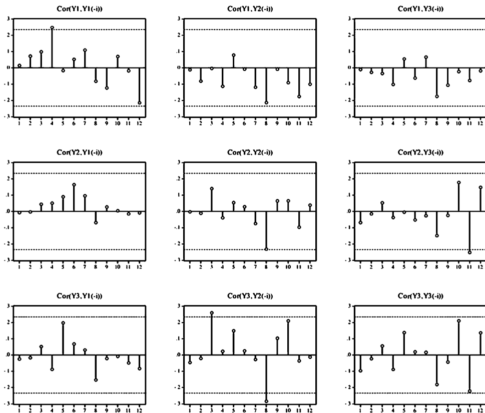
Рис. 4.1. Графики автокорреляций
