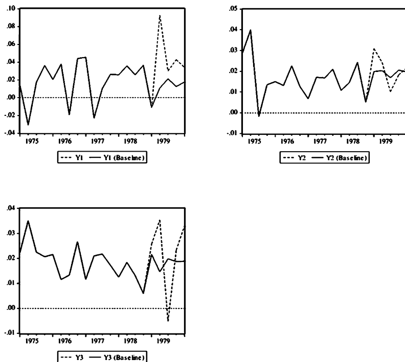
Рис. 4.2. Прогнозы VAR-модели
