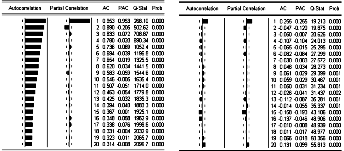
Рис. 5.2. Коррелограммы для \log(\text{price}) и d\log(\text{price})
