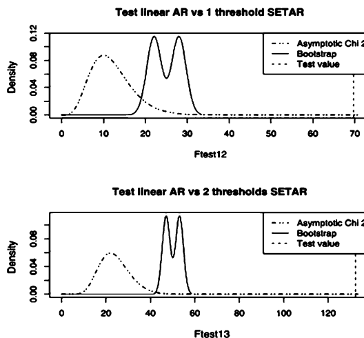
Рис. 4.12. F-тест Хансена для тестирования линейной АП-модели против СВАР(2) (SETAR)-модели. Солнечные пятна, 1700-1988 гг.
