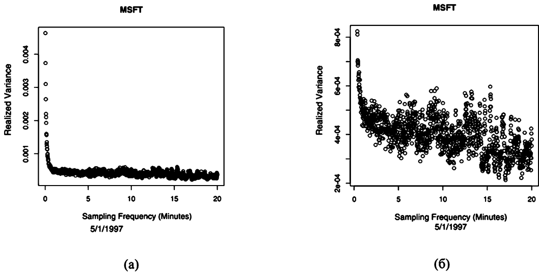
Рис. 5.11. График сигнатуры волатильности по данным за один день для MSFT, 5/1/1997
